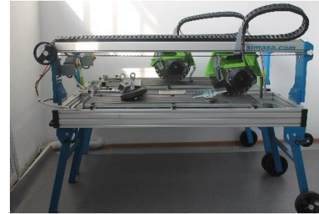
Камнерезный станок VENUS 85 MEKANO
