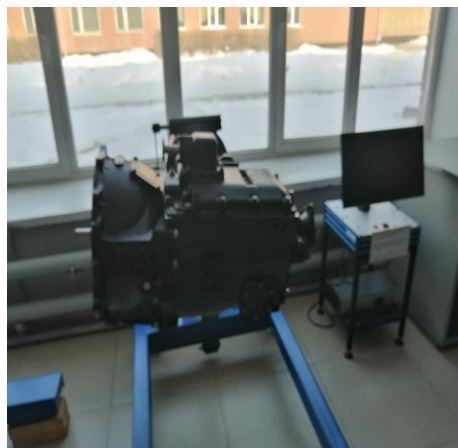
Компьютеризированный тренажерный комплекс «Механическая коробка передач» грузового автомобиля.
