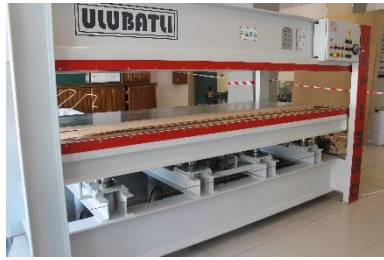
Горячий гидравлический пресс JY38410X120
