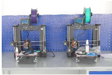
3D принтер для кровельщика I3 v2
